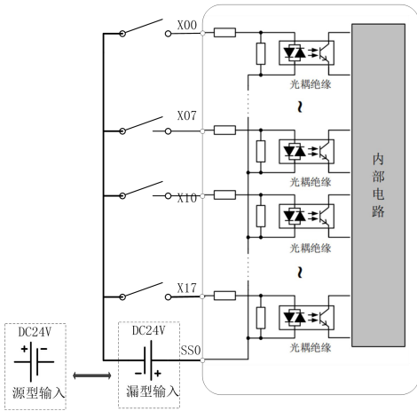
图 3-3 内部接线示意图
