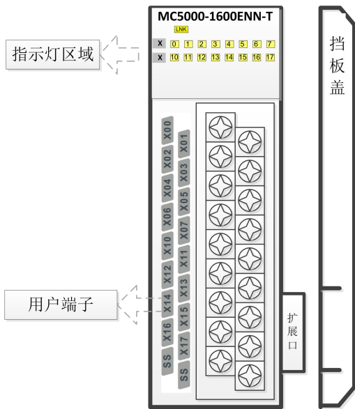
图 1-1 外观端子示意图
